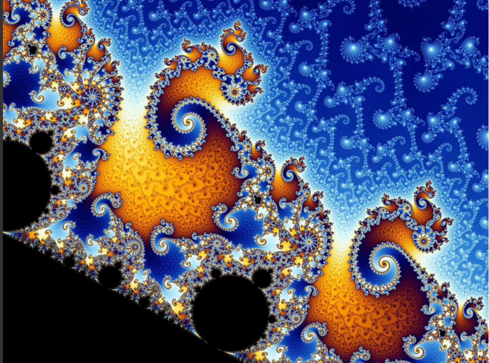
Mandelbrotova množina ↑
